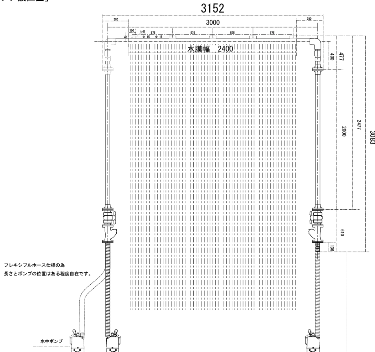
「ポンプ設置図」
